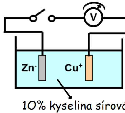
Voltův článek (asi 1V)
