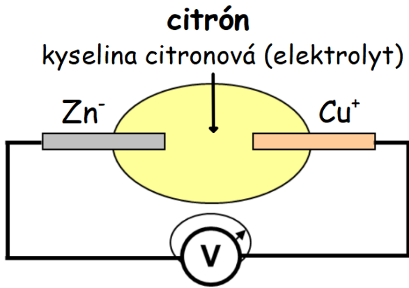
Voltův článek (asi 1V)
